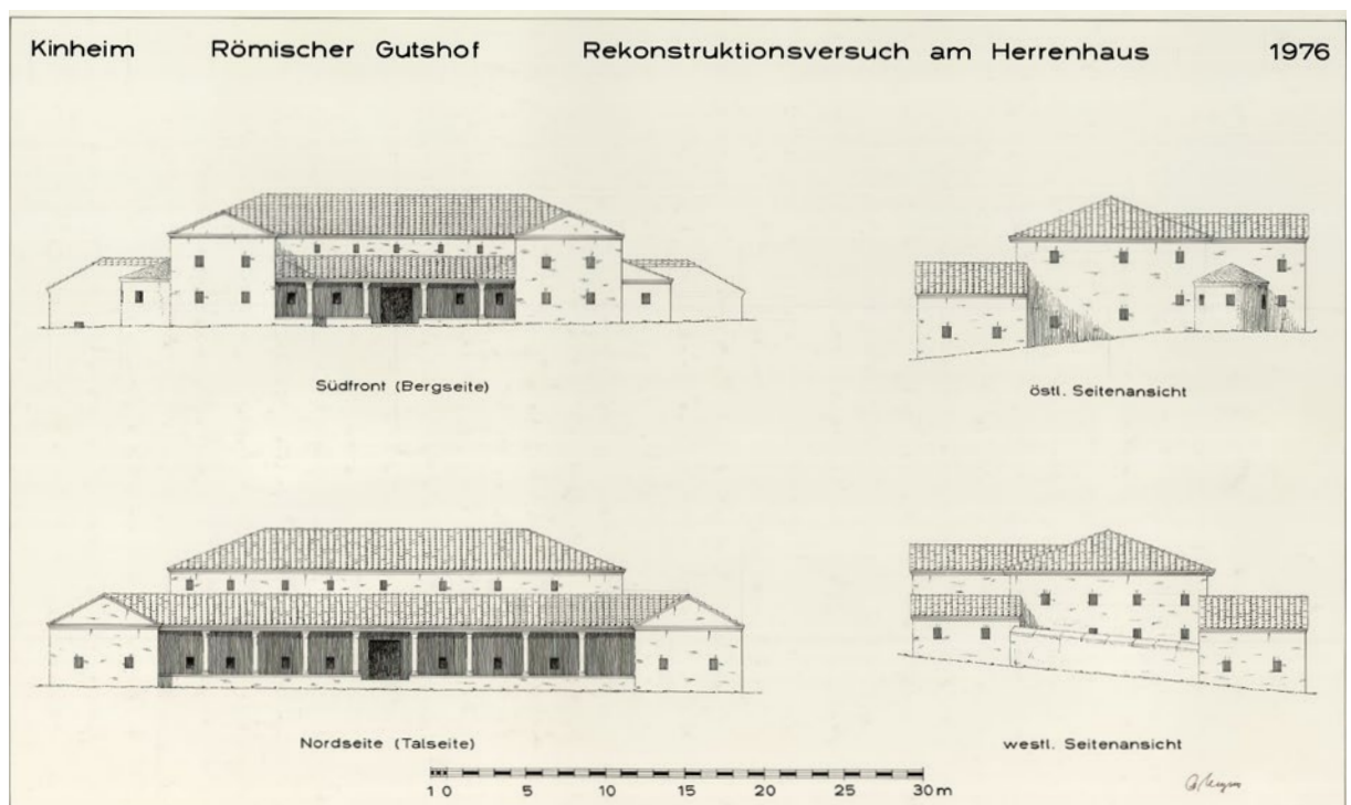
Abb. 11: Rekonstruktionsversuch Gutshof Kinheim von Adolf Neyses
