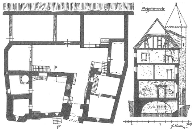
Abb. 40: Burg Grundriss
